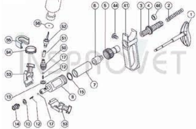
VACUNADOR SOCOREX PORTA FRASCOS
