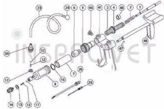
VACUNADOR SOCOREX AGUJA ASCENSION
