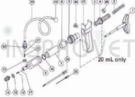
VACUNADOR SOCOREX AGUJA ASCENSION
