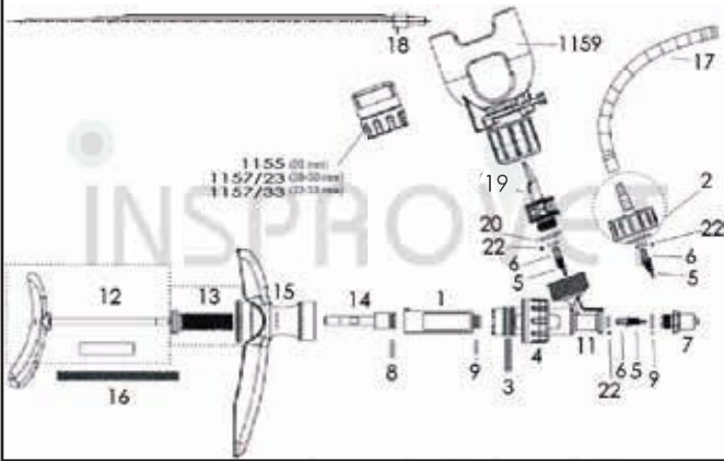
VACUNADOR MASTER LINE
